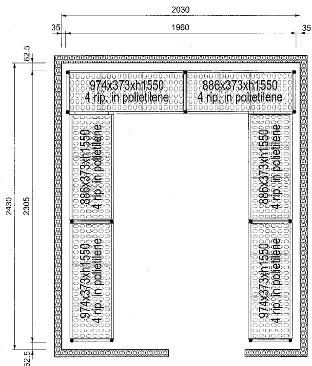
Boven aanzicht
